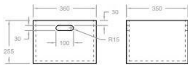
DETALLE CAJONES
